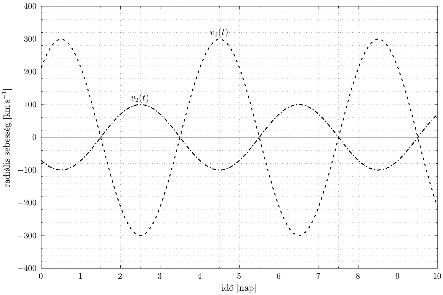
Kétvonalas spektroszkópai kettős radiálissebesség-görbéi
